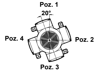
Klemens Pozisyonları Terminal Box Positions / Klemmenkasten
