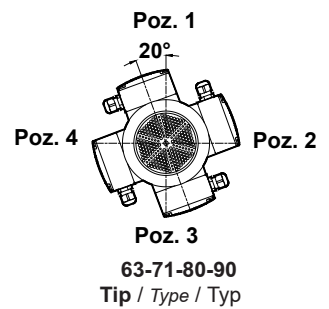
Klemens Pozisyonları Terminal Box Positions / Klemmenkasten
