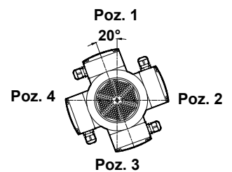
Klemens Pozisyonları Terminal Box Positions / Klemmenkasten
